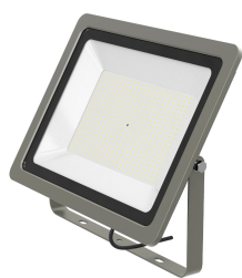
145721 LED Projecteur Gris 2.0 150W 15700lm 3000K
